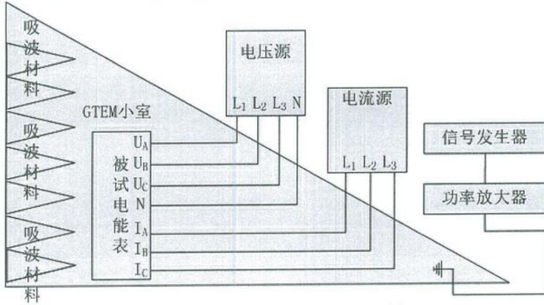
图 5 射频电磁场抗扰度试验接线布置图
