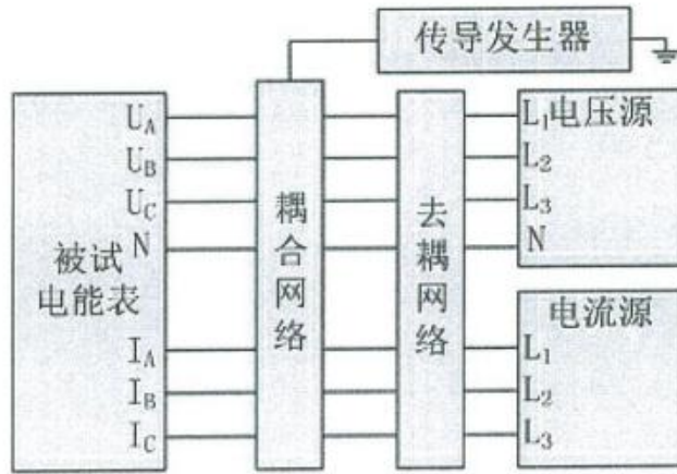
图 7 射频场感应的传导骚扰抗扰度试验接线图
