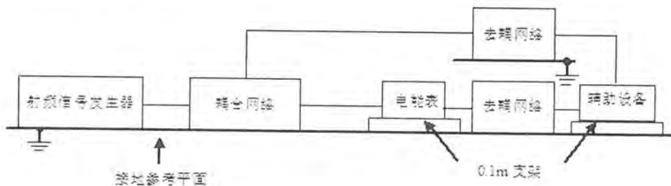
附录 4 射频场感应的传导干扰试验布置图
