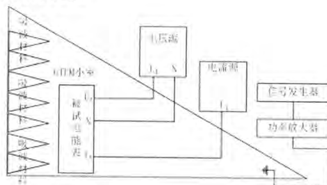
附录 7 射频电磁场试验接线布置图
