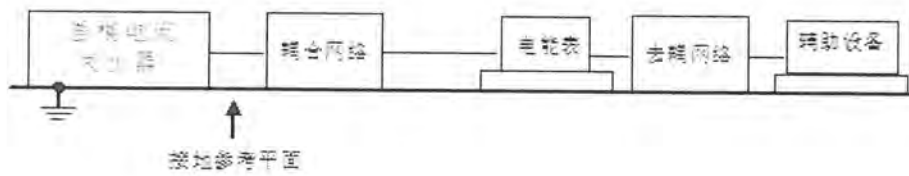
附录 14 传导差模电流干扰试验布置图
