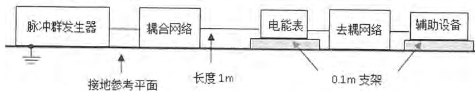
图 8 快速瞬变脉冲群试验布置图
